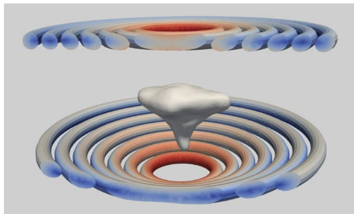
Elektromagnētiskās levitācijas tehnoloģija titāna kausēšanai (kušanas temperatūra 1670°C) un liešanai.
