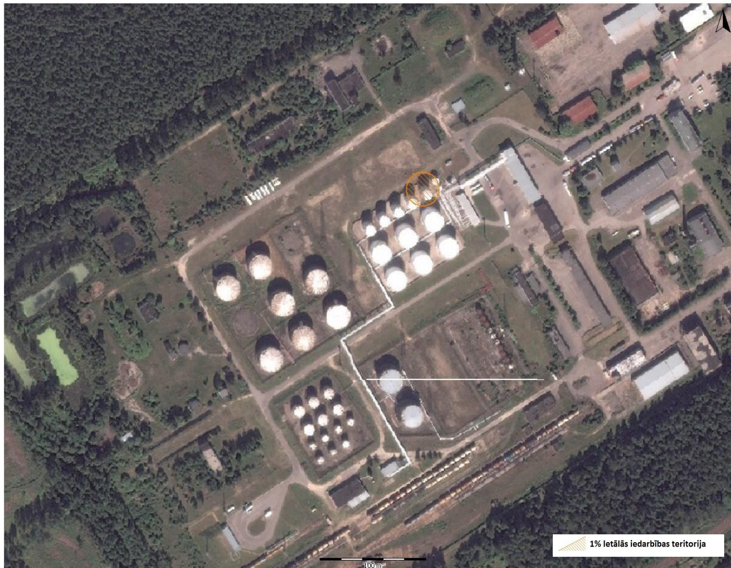
2.15. attēls. Maksimālā 1% letālās iedarbības zona etanola rezervuāra tūlītējas izplūdes un ugunsgrēka gadījumā (piemērs, attēlota rezervuāra Nr. VI-11 avārija)
