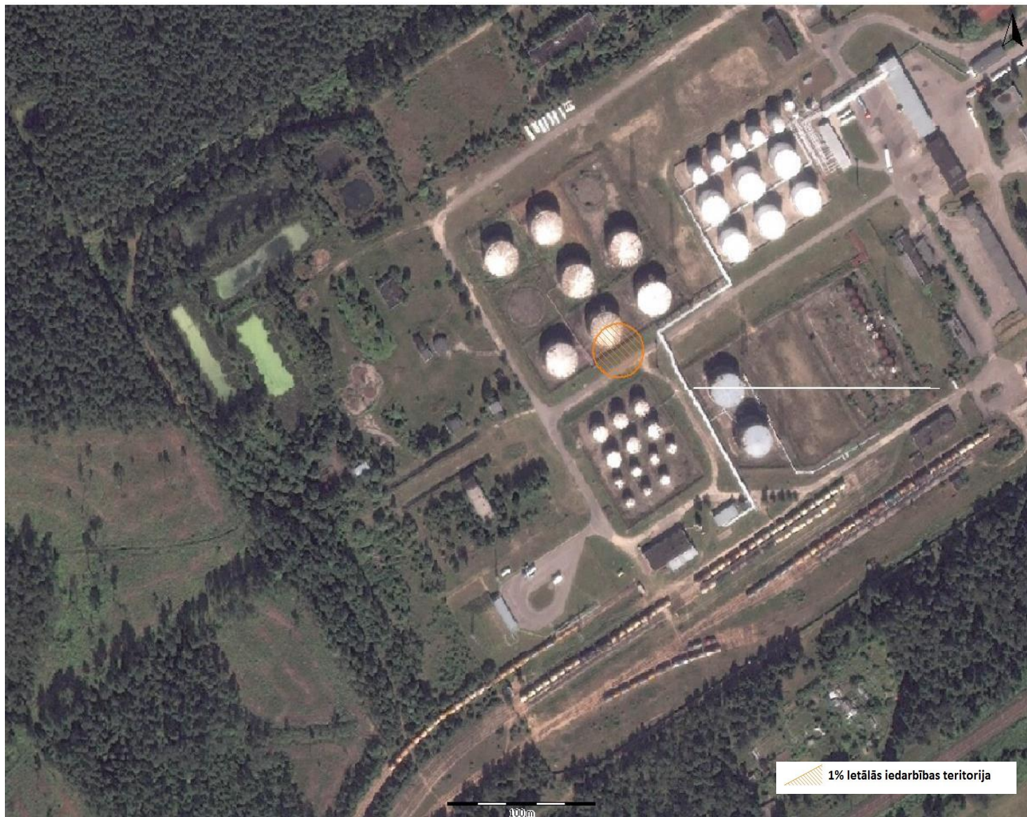
2.12 attēls. Maksimālā 1% letālās iedarbības zona peļķes ugunsgrēka gadījumā sūkņu stacijā Nr. 5 (piemērs)
