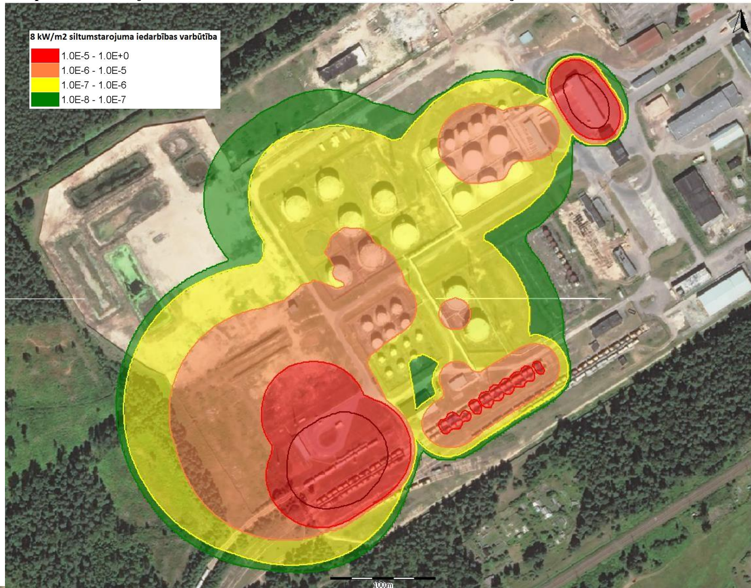
4.22.attēls. Iespējamo avārijas scenāriju radītā siltumstarojuma ar 8 kW/m 2 apdraudētā teritorija un šī apdraudējuma varbūtība
