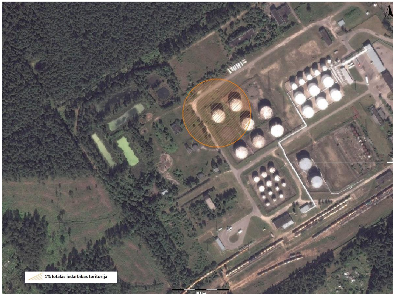
2.16. attēls. Maksimālā 1% letālās iedarbības zona dīzeļdegvielas rezervuāra tūlītējas izplūdes un ugunsgrēka gadījumā (piemērs, attēlota rezervuāra Nr. 1 avārija)
