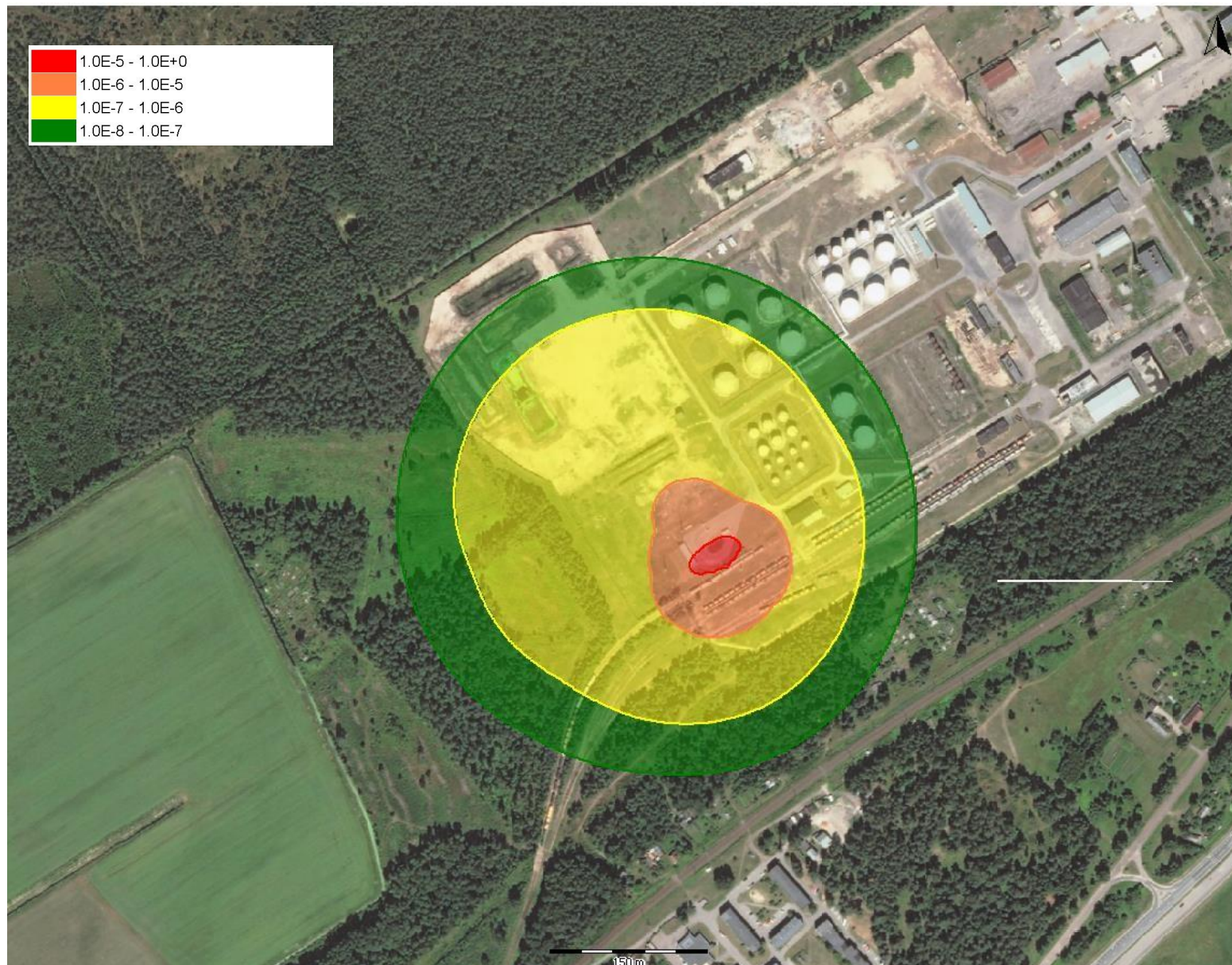
2.23.attēls. Iespējamo avārijas scenāriju radītā pārspiediena 0,1\text{bar} apdraudētā teritorija un šī apdraudējuma varbūtība
