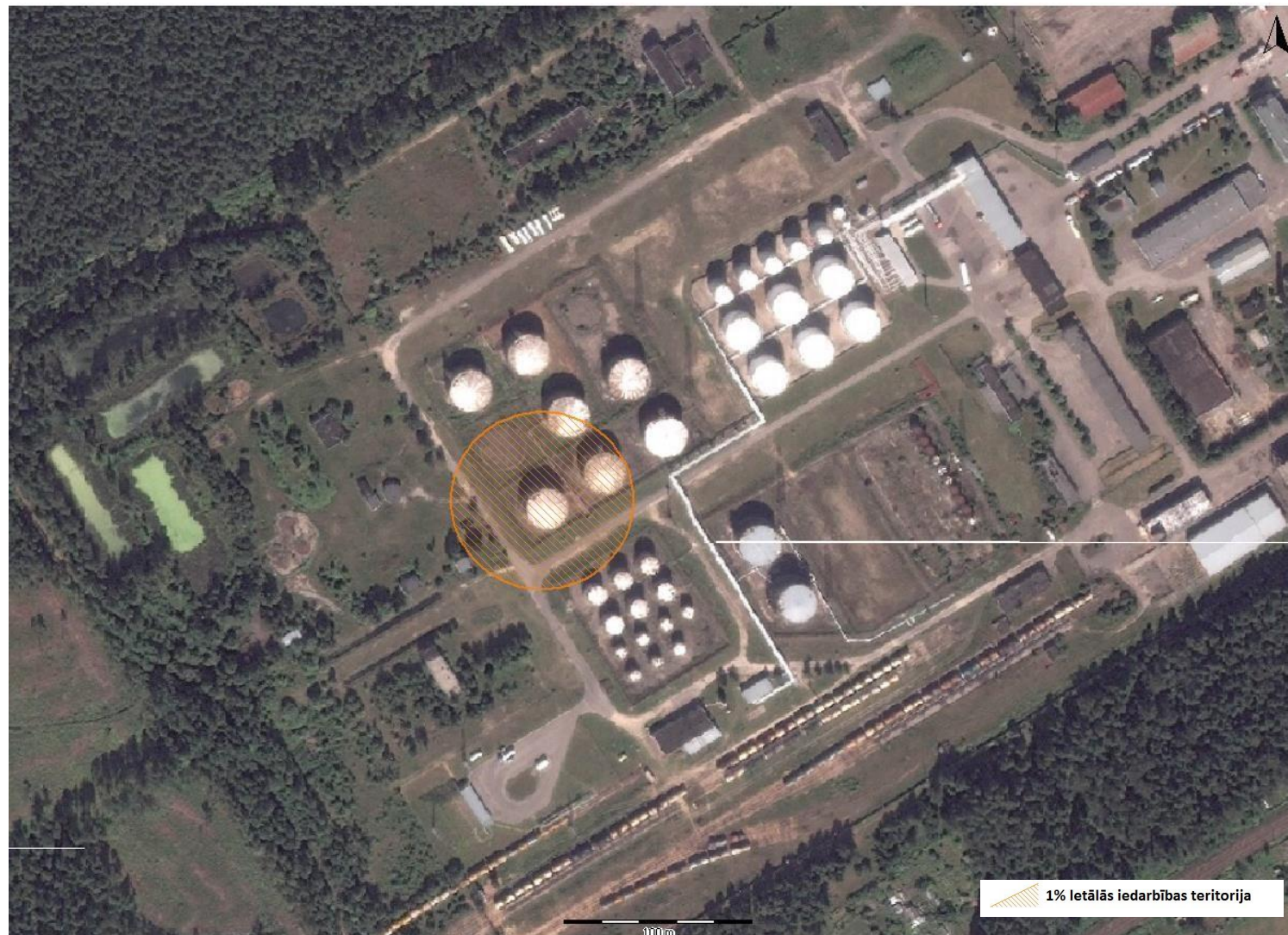
2.18. attēls. Maksimālā 1% letālās iedarbības zona benzīna rezervuāra tūlītējas izplūdes un ugunsgrēka gadījumā (piemērs, attēlota rezervuāra Nr. 12 avārija)
