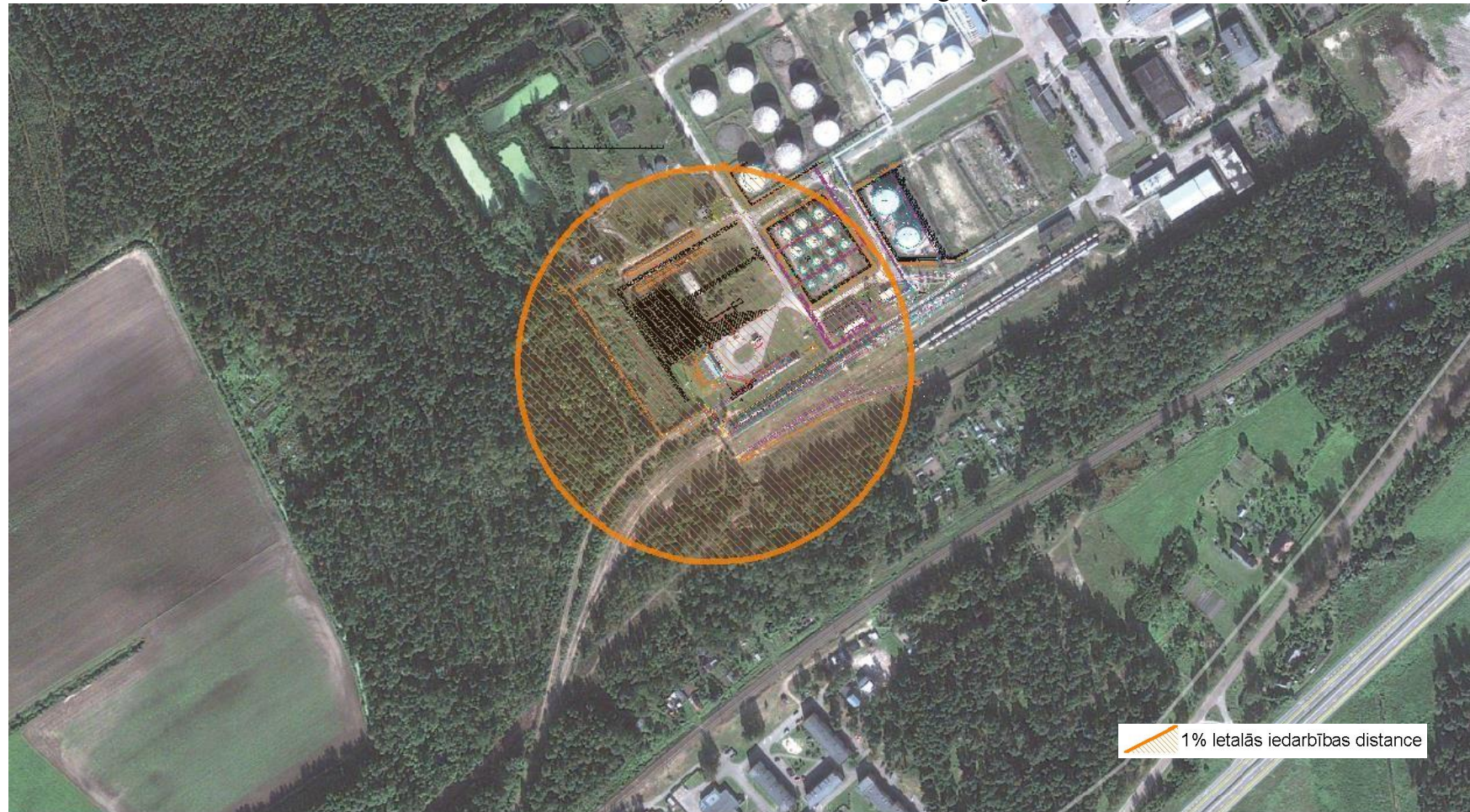
2.1. attēls. Maksimālās 1% letālās iedarbības zona vienas dzelzceļa cisternas BLEVE gadījumā dzelzceļa cisternu noliešanas estakādē
