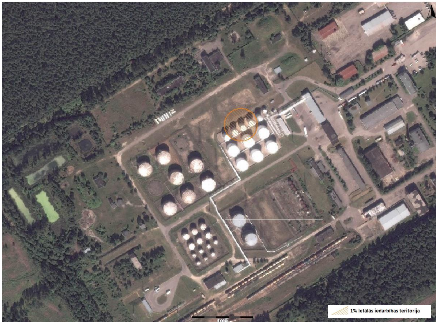
2.14. attēls. Maksimālā 1% letālās iedarbības zona benzīna rezervuāra tūlītējas izplūdes un ugunsgrēka gadījumā (piemērs, rezervuārs Nr. VI-9)
