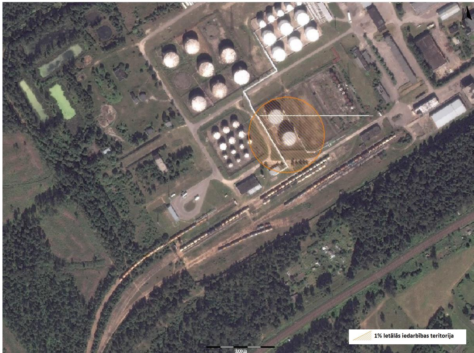
2.20.attēls. Maksimālā 1% letālās iedarbības zona dīzeļdegvielas rezervuāra tūlītējas izplūdes un ugunsgrēka gadījumā (piemērs, rezervuāra Nr. 31 sabrukums)
